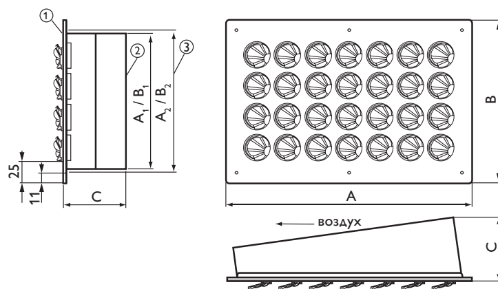
1 – Воздухораспределитель; 2 – Рассекатель; 3 – Размер проема в воздуховоде.
