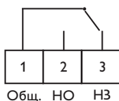
Схема подключения
