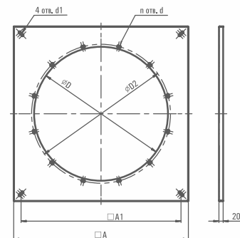
ИСПОЛНЕНИЕ ПЕРЕХОДНИК ПЛОСКИЙ (ПеП)
