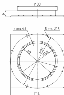
ИСПОЛНЕНИЕ ПЕРЕХОДНИК КРЫШНЫЙ (ПеК)
