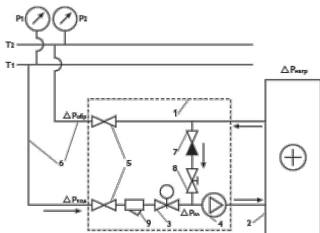
С двухходовым регулирующим вентилем
