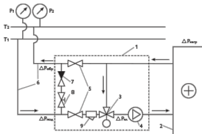
С трехходовым регулирующим вентилем
